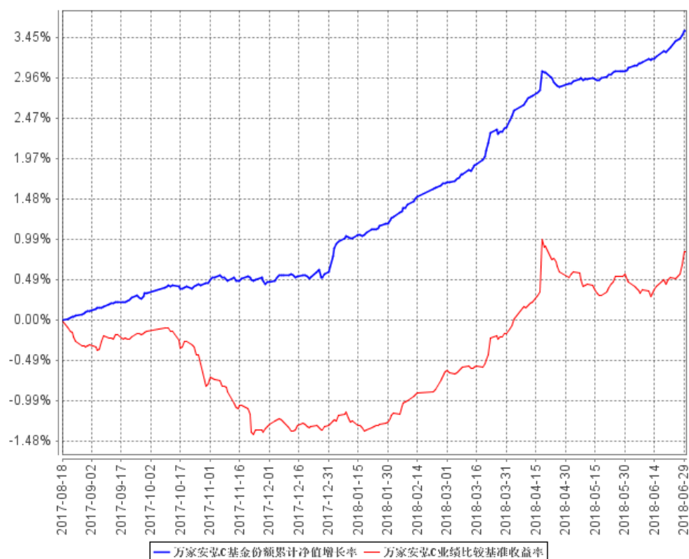
万家安弘C基金份额累计净值增长率与同期业绩比较基准收益率的历史走势对比图
